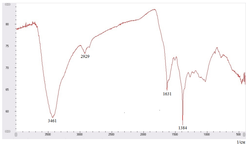
Рис. 4. ИК-спектр гидрогеля ОГЛ и \text{Pb}(\text{NO}_3)_2
