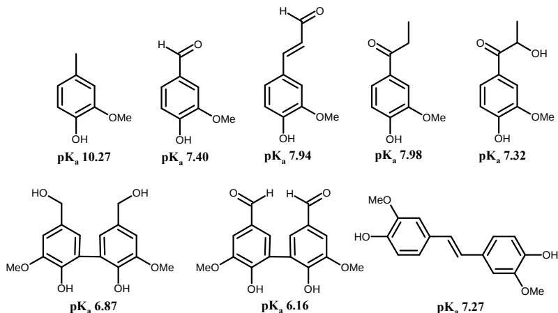
Рис. 10. Значения \text{pK}_a модельных соединений лигнина
