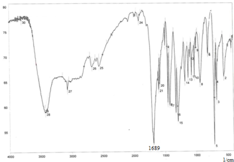
Рис. 5. ИК-спектр бензойной кислоты
