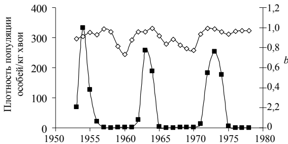
Рис. 2. Соотношения между плотностью популяций Zeiraphera griseana Hübner в лиственничных лесах Альп (1) и коэффициентом b (2) рангового распределения видов в сообществе (—■)— 1; (---◇)— 2
